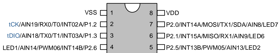
SC92F5310 管脚配置图 适用于 SOP8 封装
