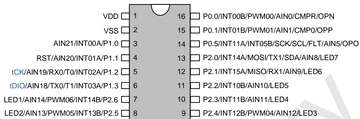
SC92F5311 管脚配置图 适用于 SOP16 封装
