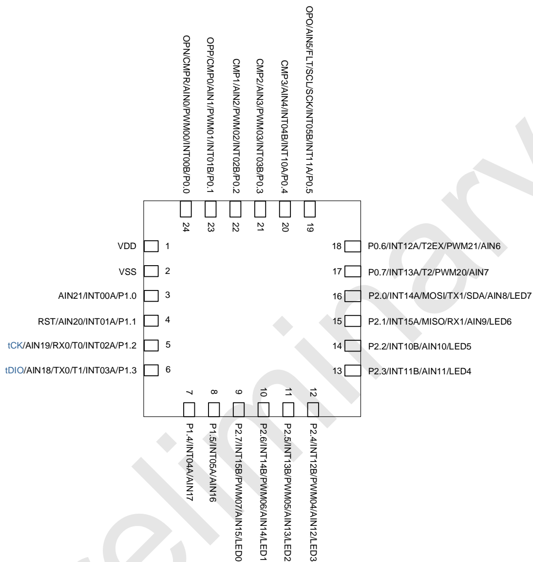
SC92F5319 管脚配置图 适用于 QFN24 封装
